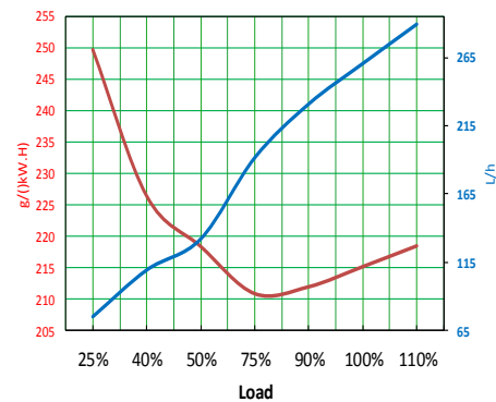
12M26G910/6e2-1014kW/1800rpm
